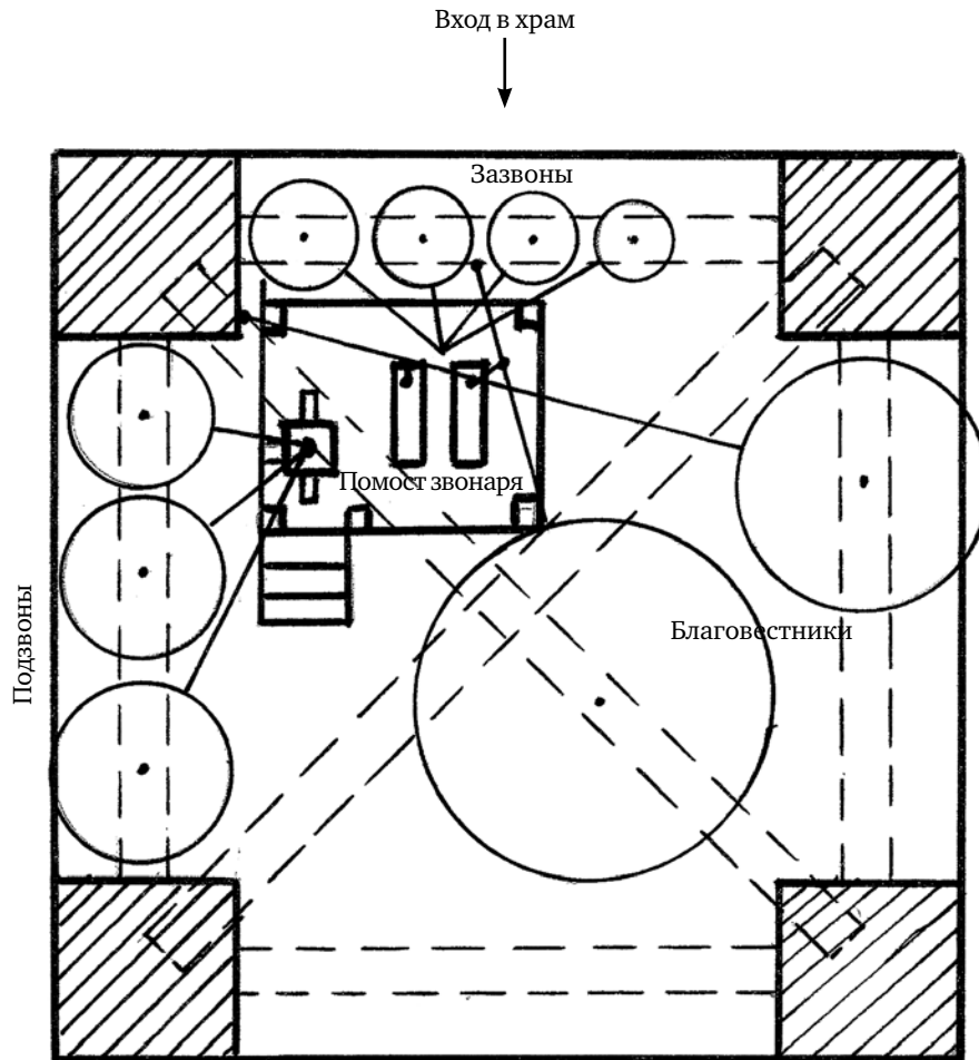
Вариант правильного размещения колоколов и тяг для управления ими в храме «Иже под колоколы» (квадратный ярус звона). Схема предоставлена Московским колокольным центром
