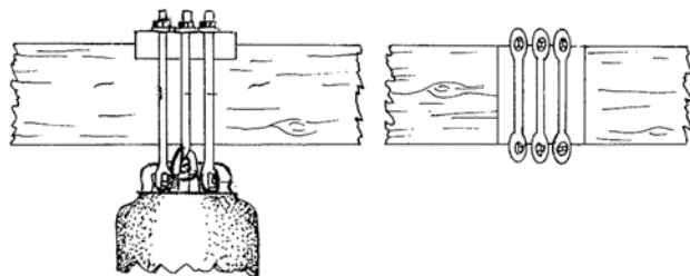
Рис. 1. Правильная установка хомутов на балку
