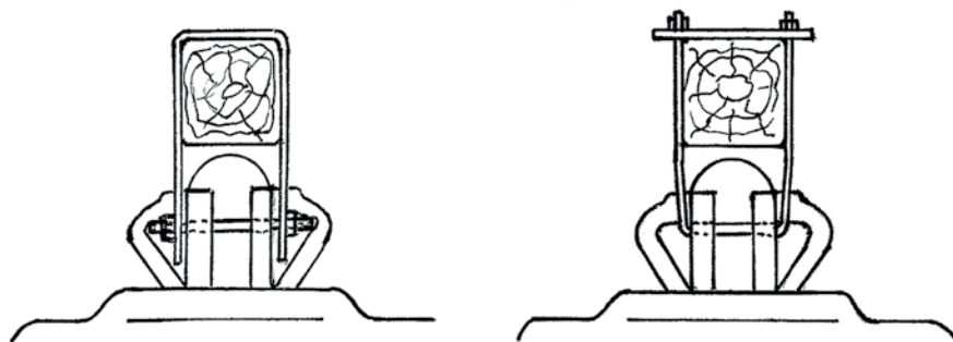
Рис. 2. Пропуск опорной шпильки в сквозные отверстия хомутов и уши колокола
