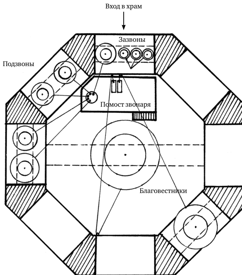
Вариант правильного размещения колоколов и тяг для управления ими в храме «Иже под колоколы» (восьмигранный шатер). Схема предоставлена Московским колокольным центром
