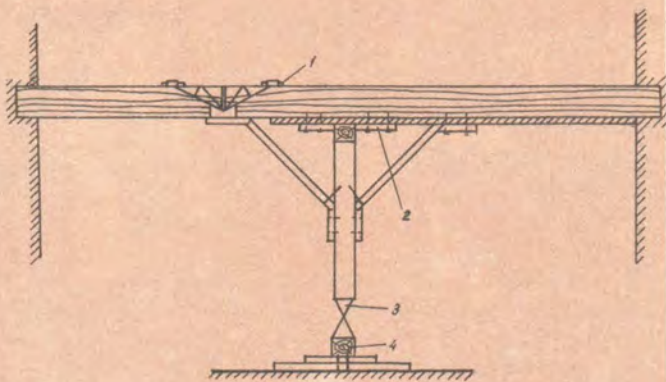
Рис. 2. Крепление опорных лесов при вывешивании перекрытий:
