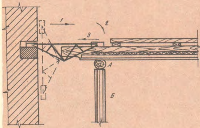
Рис. 1. Установка концевой протеза: 1, 2 и 3 — последовательность операций
