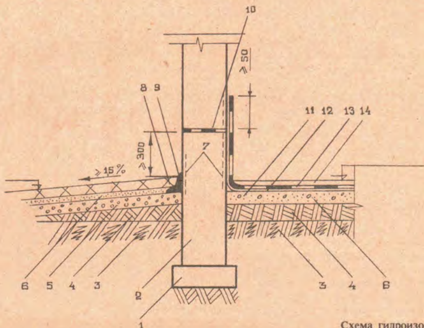
Схема гидроизоляции
